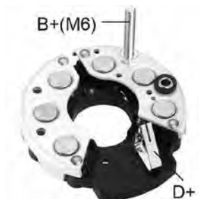
RB-12H *90mm OD *6-35 Amp Diodes
